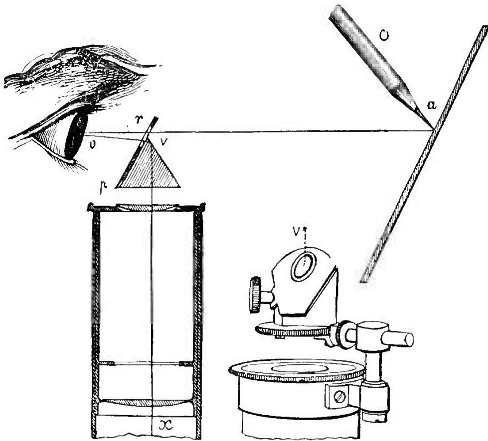
Fig. 143. — Chambre claire.
