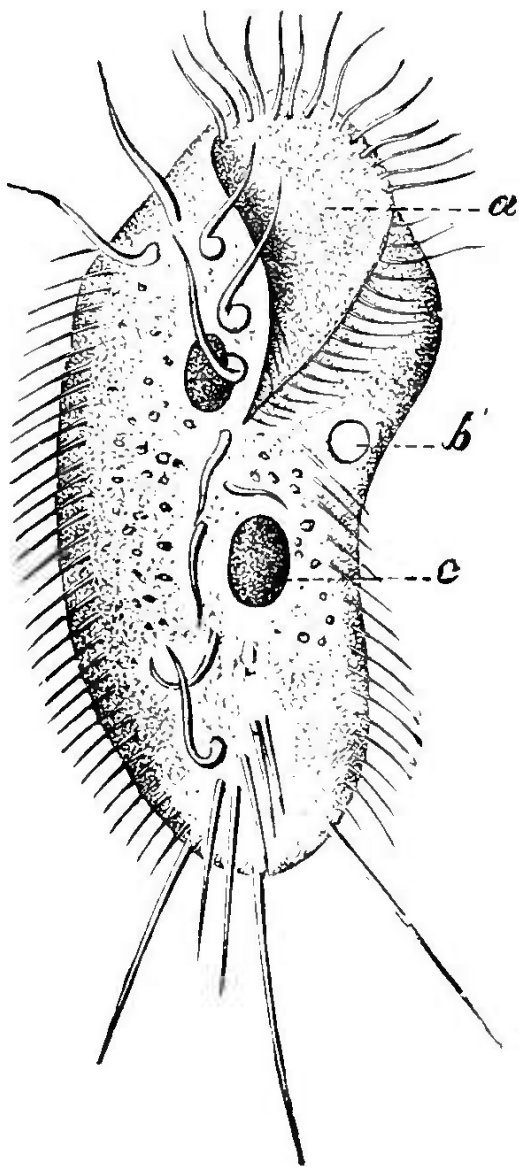
Fig. 58. — Stylonichia mytilus .
