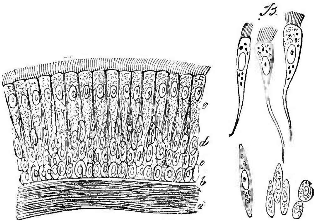
Fig. 33. — Épithélium vibratile.
