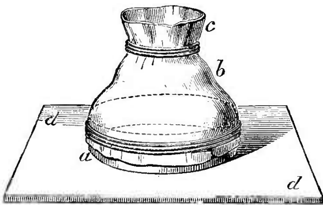
Fig. 144. — Chambre humide.
