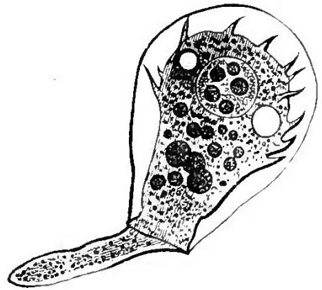
Fig. 117. — Hyalosphaeria lata .
