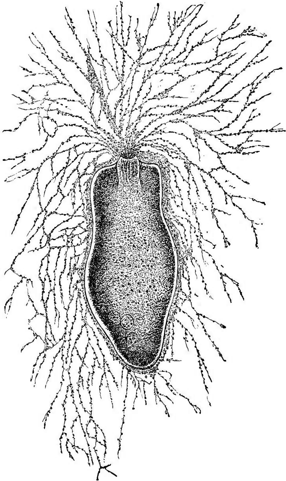
Fig. 59. — Gromia oviformis .
