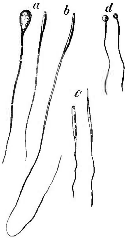
Fig. 37. — Spermatozoïdes.
