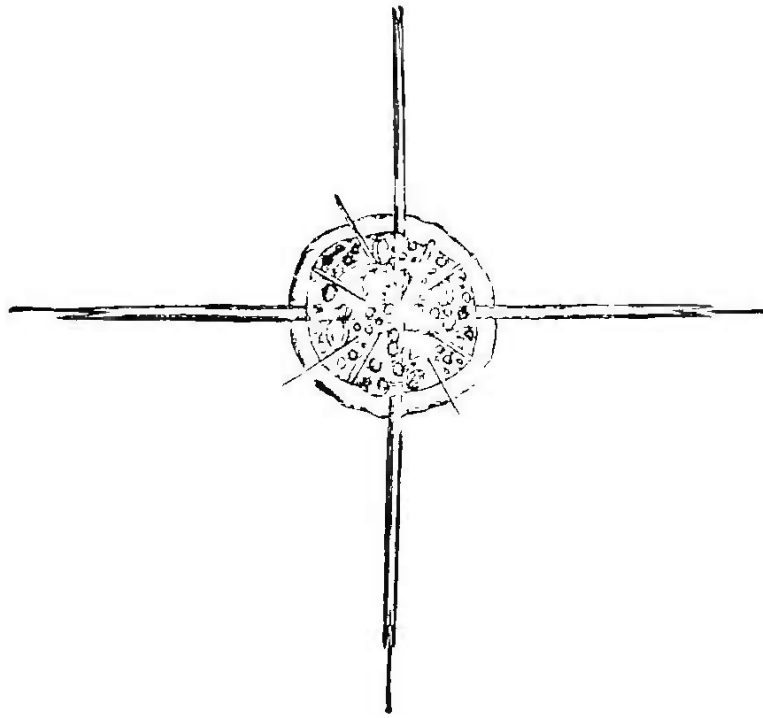
Fig. 123. — Acanthometra pallida .
