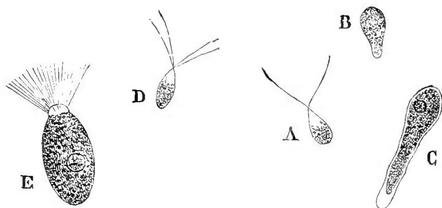
Fig. 44. — Zoospores d'Algues.
