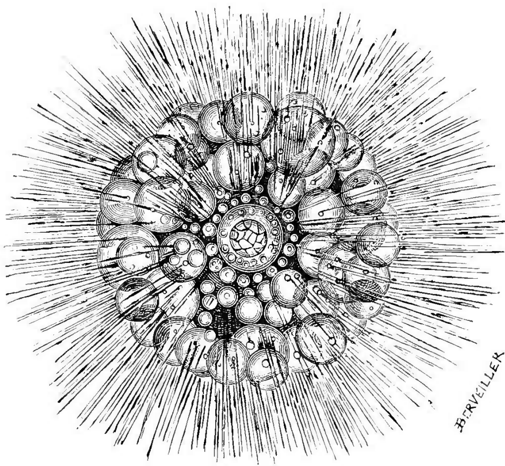
Fig. 70. — Thalassicole pélagique.
