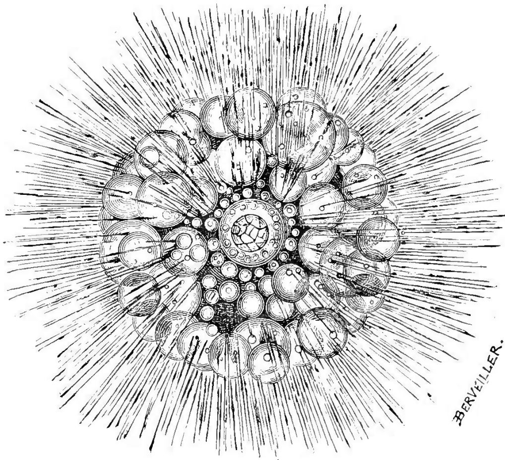
Fig. 124. — Clathruline élégante.
