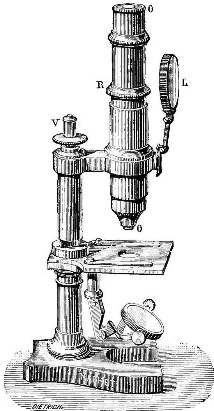
Fig. 440. — Microscope (Modèle Nachet).
