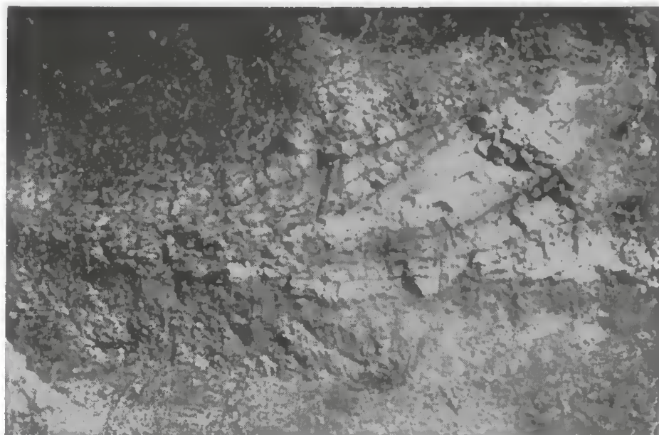
FOTO 3 — Estrutura deltáica amostra D-1
