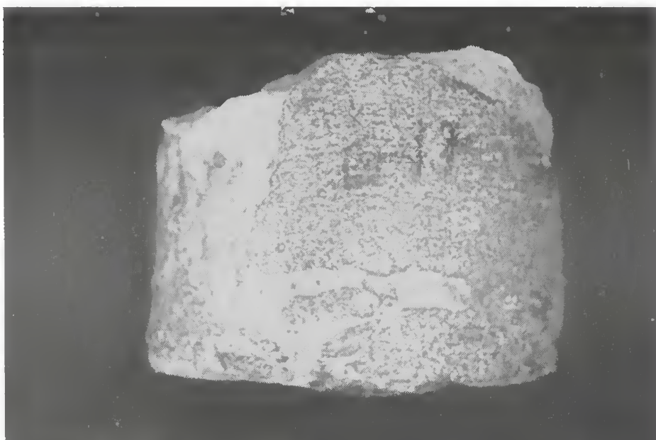
FOTO 5 — Membro Itaqueri (conglomerado basal) — Amostra G-17
