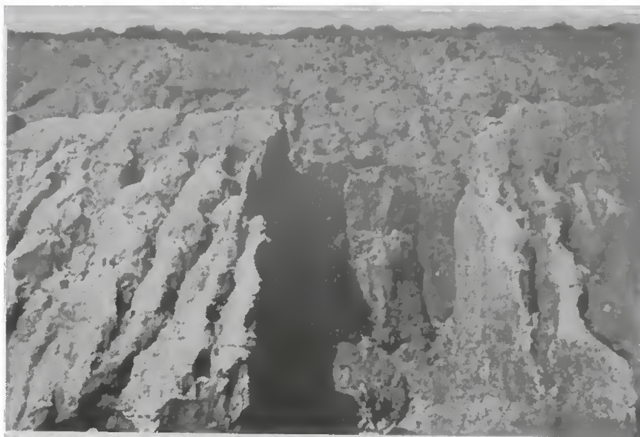
FOTO 11 — Erosão no membro Bauru em rochas sem cimento calcáreo. Corte E. F. S. Km 273. Entre Botucatu e Rubião Júnior.
