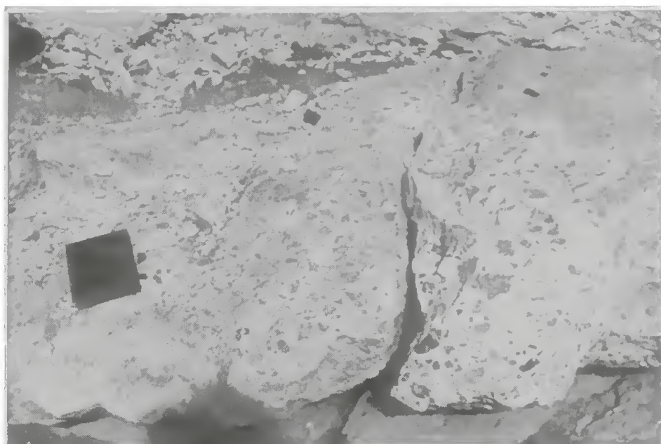
FOTO 7 — Membro Itaquerí — Altitude 848 m. Corte Km 272,150 da E.F.S. Entre Botucatu e Rubião Júnior.
