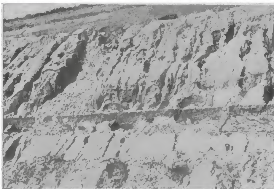
FOTO 8 — Facies argilítico no membro arenito Bauru. Corte Km 272,700 da E.F.S. Altitude 870 m.
