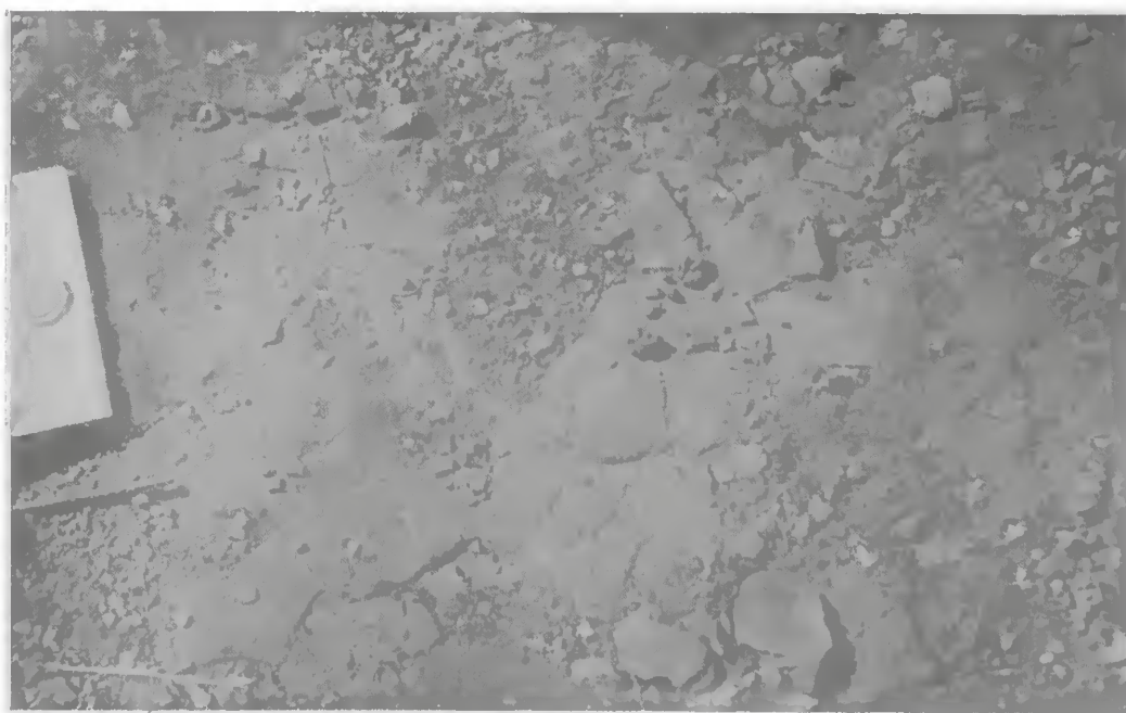
FOTO 12 — Superfície da lava pré-série Bauru (recentemente descoberta).
